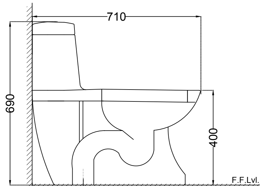
220 S-TRAP
